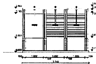
РАЗРЕЗ 1-1 М 1:50
