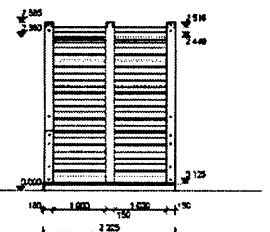
РАЗРЕЗ 2-2 М 1:50
