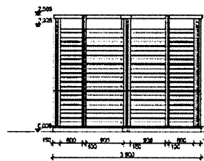
РАЗРЕЗ 1-1 М 1:50
