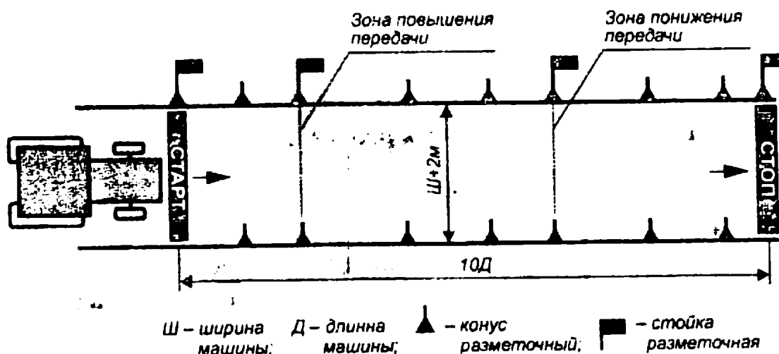
Рис. 2. Разгон-торможение
