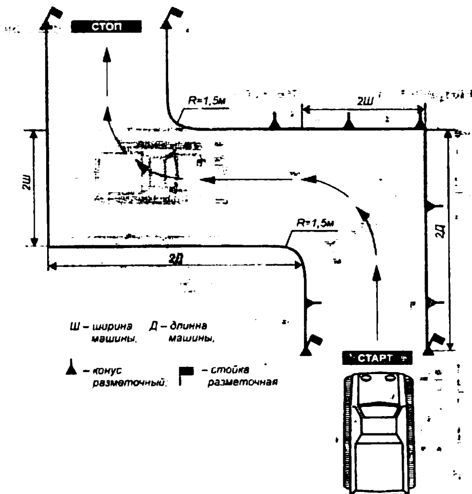
Рис. 14. Повороты на 90°
