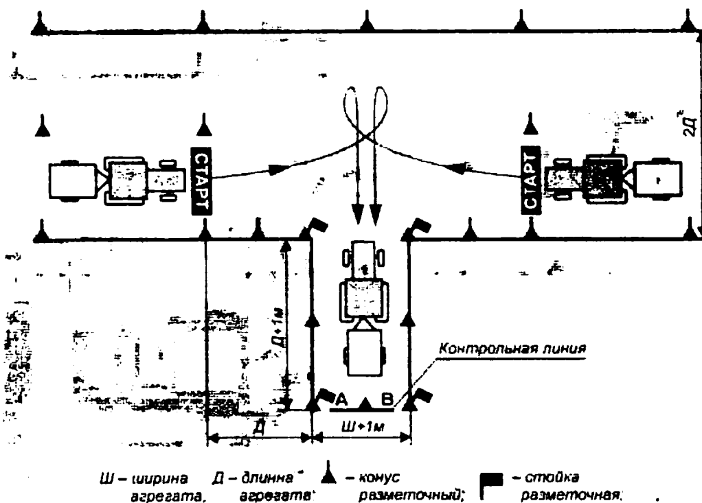
Рис. 7. Движение задним ходом, въезд в "бок" в агрегате с прицепом
