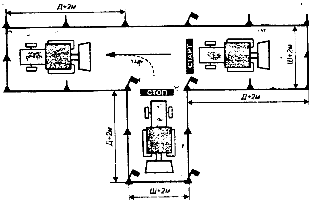
Рис. 9. Агрегатирование с навесной машиной или прицепом
