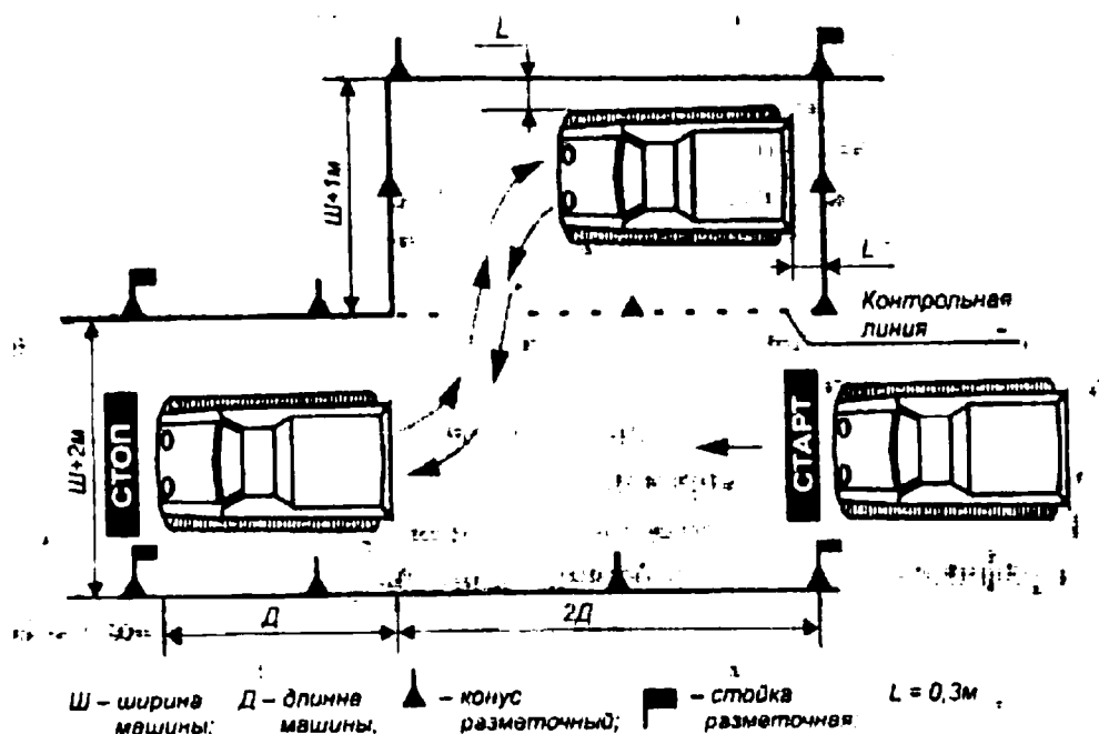
Рис. 15. Парковка СМ задним ходом и выезд с парковочного места, параллельная парковка
