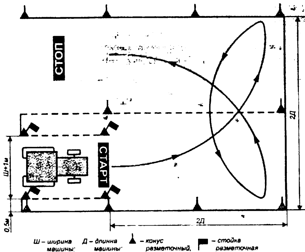
Рис. 5. Разворот маневрирование в ограниченном пространстве
