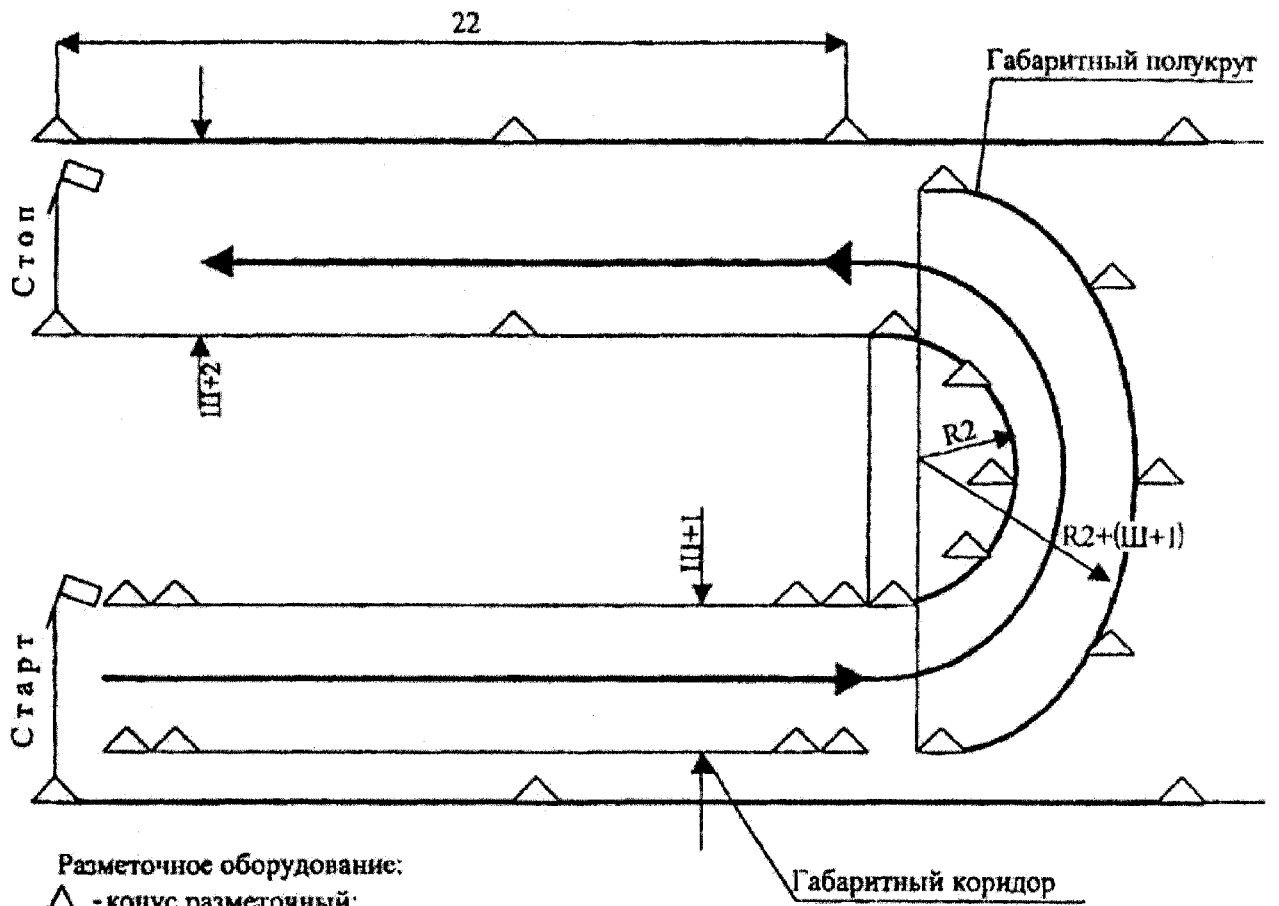
Схема 2. Габаритный коридор, габаритный полукруг
