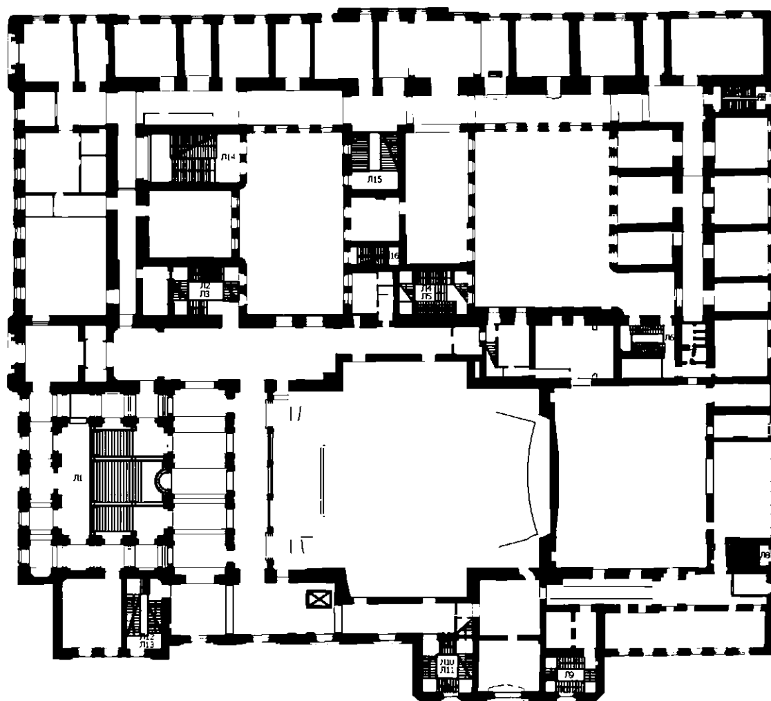
План 2 этажа с указанием местоположения лестниц
