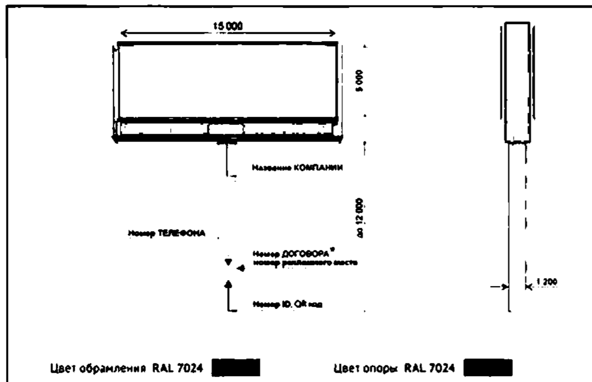
РАЗМЕРЫ
