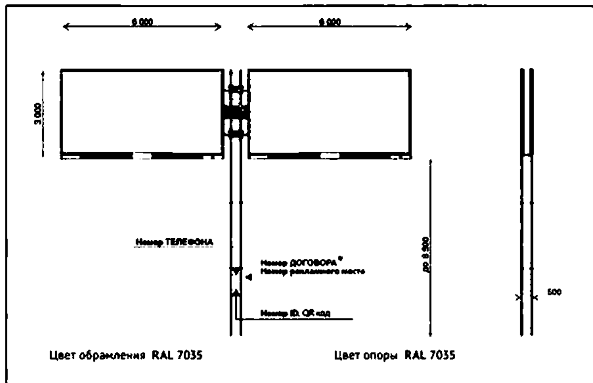
РАЗМЕРЫ МАРКИРОВКИ
