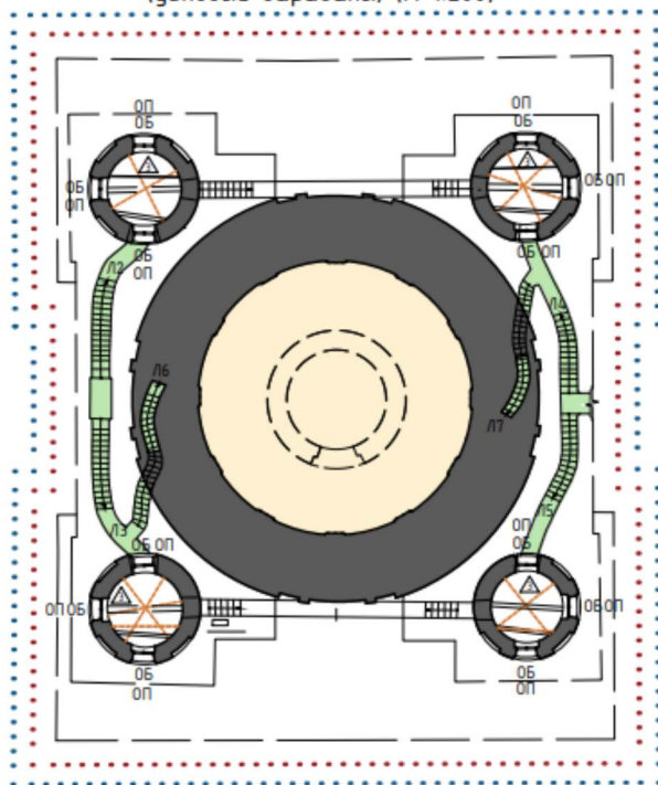
План на отметке +15,950 (угловые барабаны) (М 1:200)
