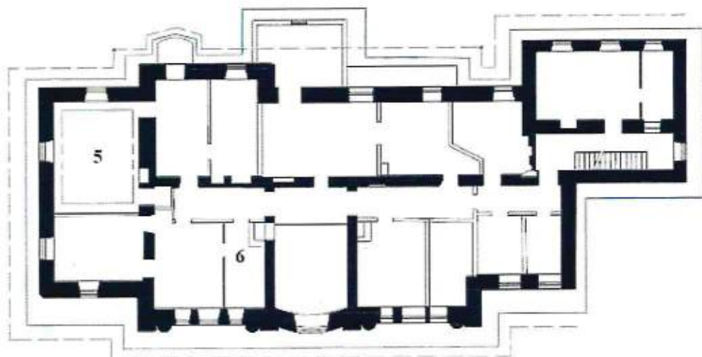
План второго этажа
