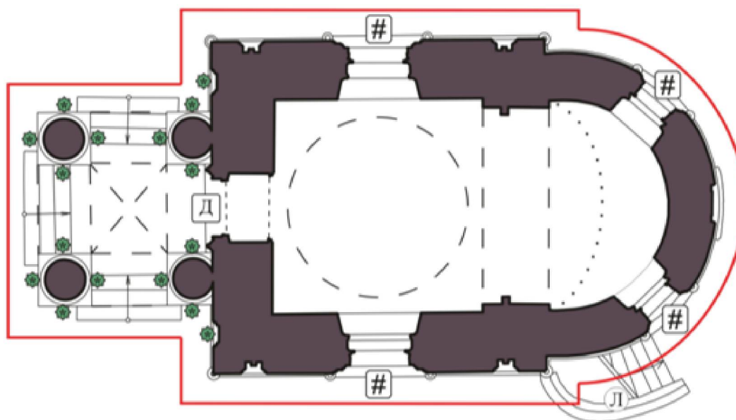
2. План первого этажа
