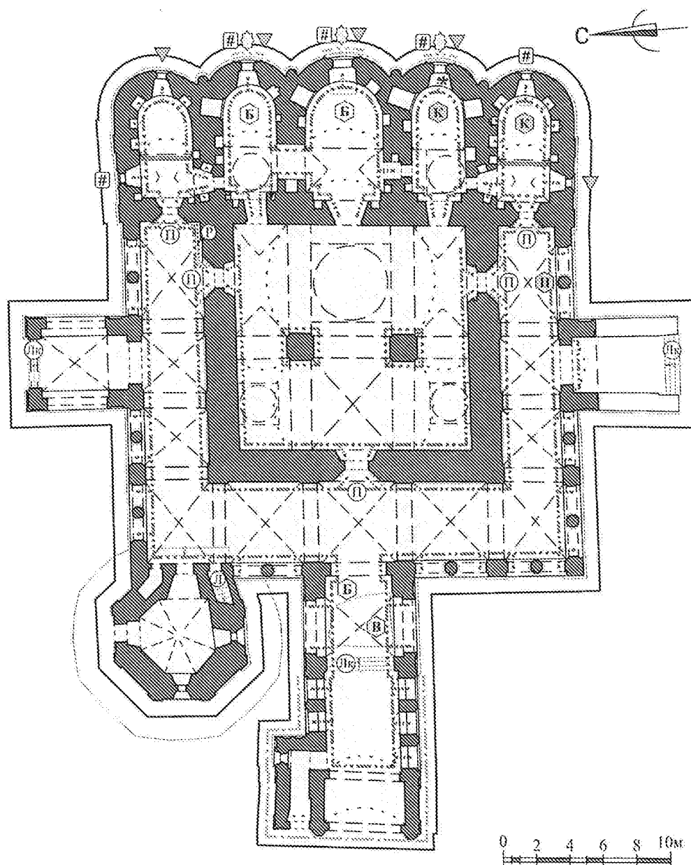
План 1 этажа
