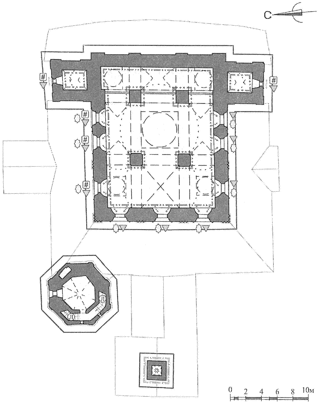
План на уровне окон второго света и второго яруса колокольни
