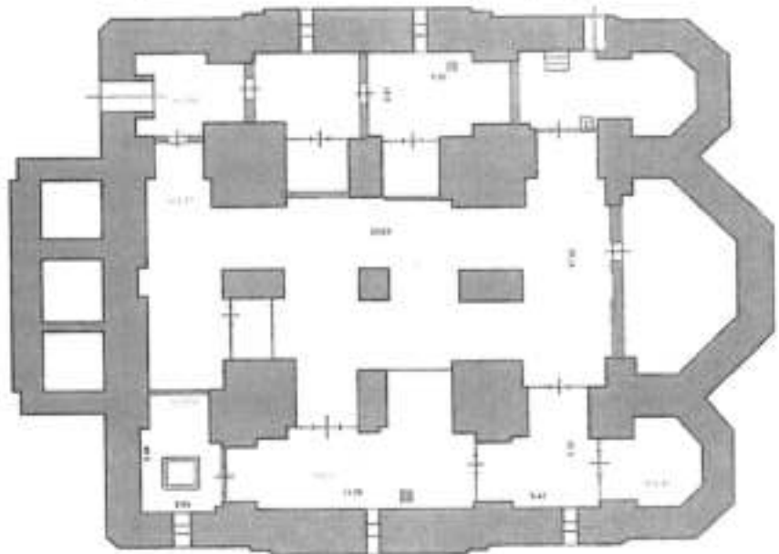
План подвала
