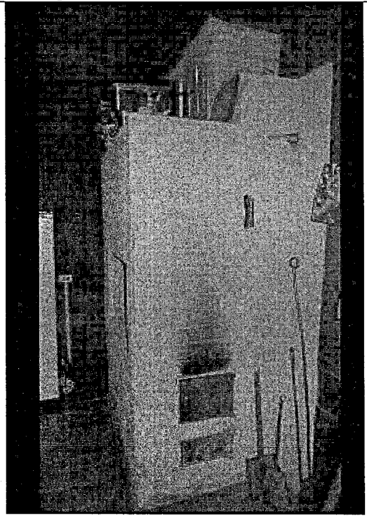
Фото 7. Средстенная печь-камин: затопочная часть с варочной поверхностью
