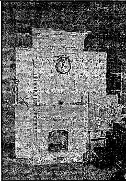
Фото 6. Средстенная печь-камин
