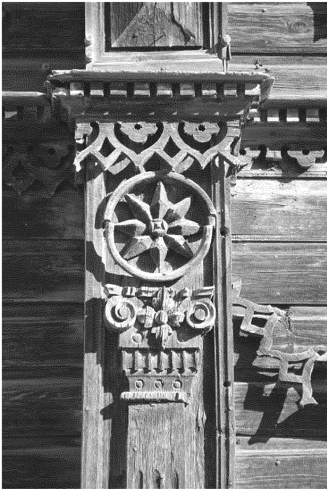
Видовая точка № 6. Фрагмент декора лопатки главного фасада (1 этаж)
