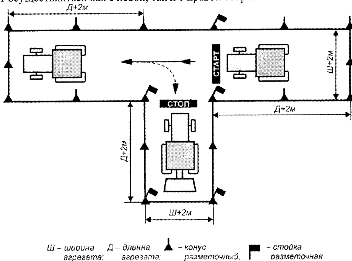
Рис. 6. Агрегатирование самоходной машины с навесной машиной
