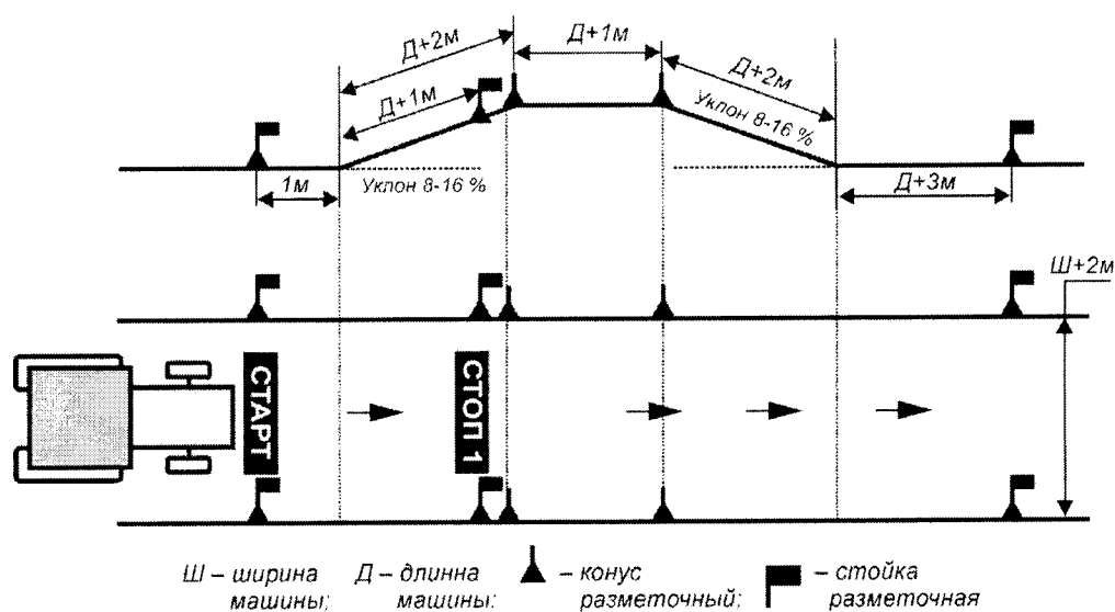
Рис. 1. Начало движения с места на подъеме
