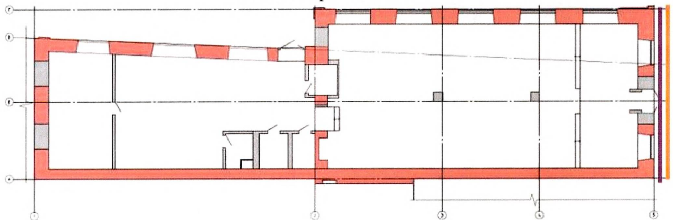
План первого этажа
