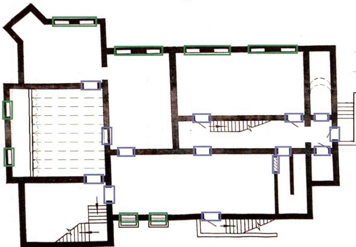
План подвала
