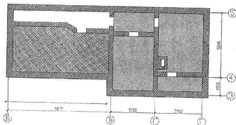
План подвала
