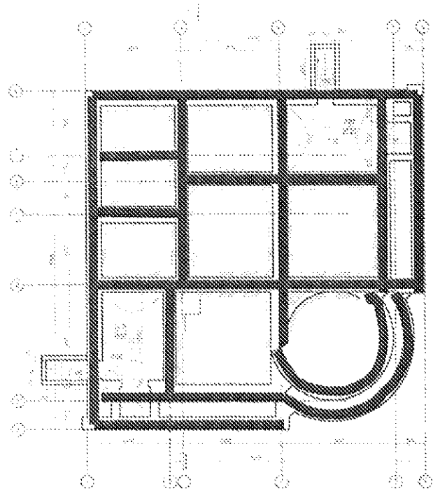
План подвала
