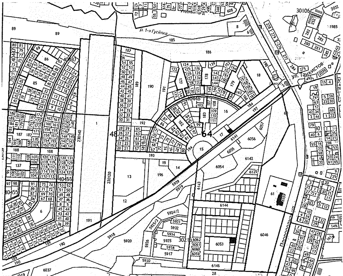
Схема 26. Объект «Газопровод высокого и низкого давления, 2 ПРГ, земли НИИ Юго-Востока, г. Саратов Саратовской области»
