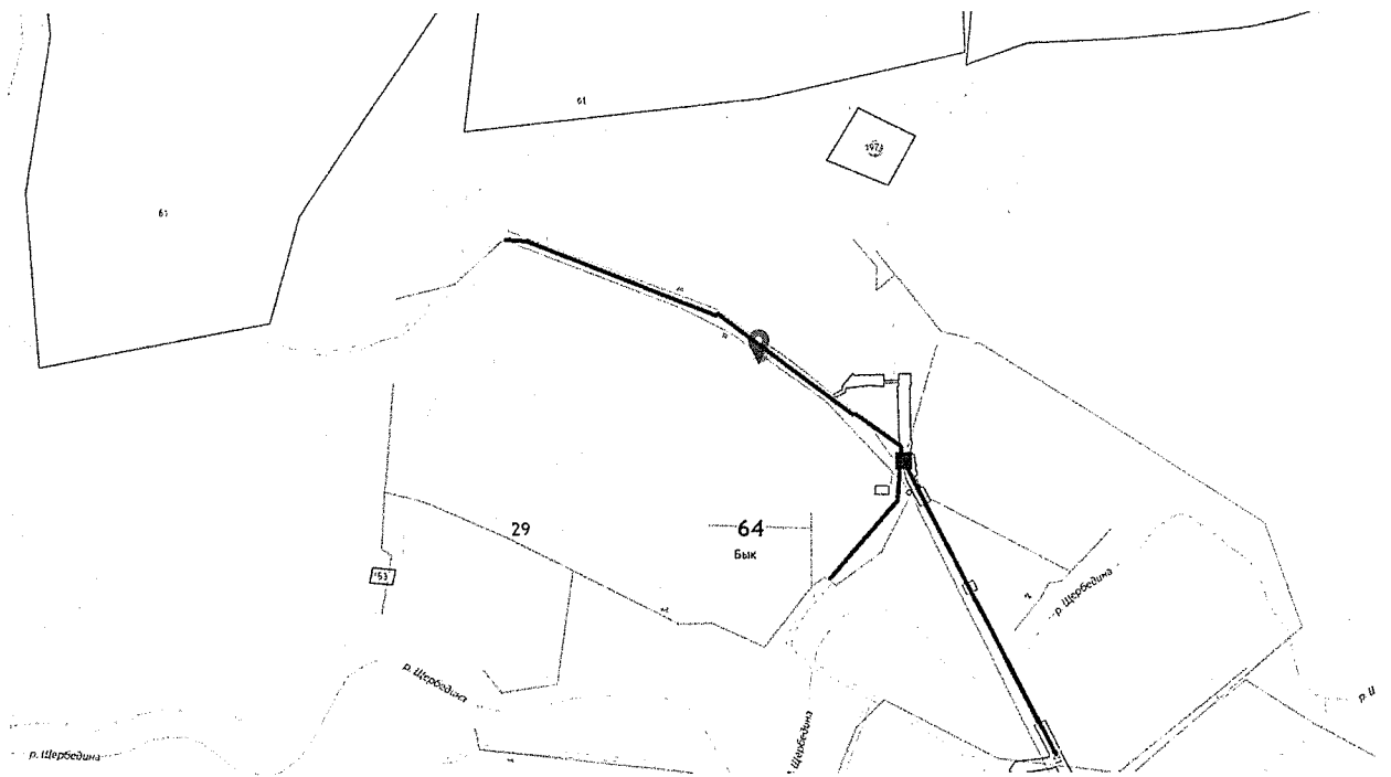
Схема 1. Объект «Распределительный газопровод с. Бык, Романовский район Саратовской области»
