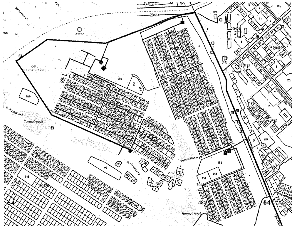
Схема 26. Объект «Газопровод высокого и низкого давления, 2 ПРГ, земли НИИ Юго-Востока, г. Саратов Саратовской области»
