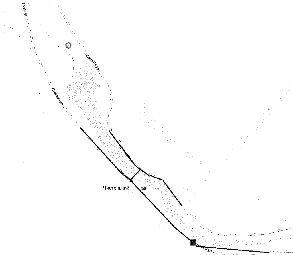
Схема 9. Объект «Распределительный газопровод в п. Чистенький, Аркадакского район Саратовской области»
