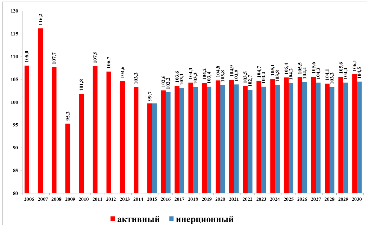
Рисунок 1. Годовые прогнозные темпы роста ВРП Пензенской области в активном и инерционном вариантах сценария (2006–2030 годы, в процентах к предыдущему году)
