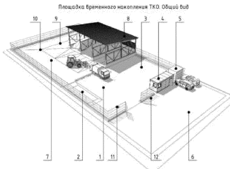
Экспликация зон и сооружений площадки временного накопления ТКО
