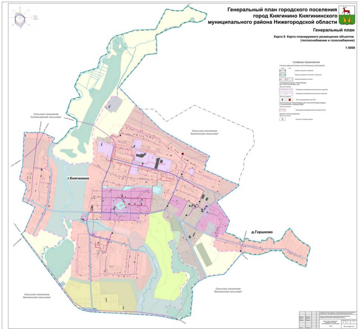
Карта 8. Карта планируемого размещения объектов (теплоснабжение и газоснабжение)
