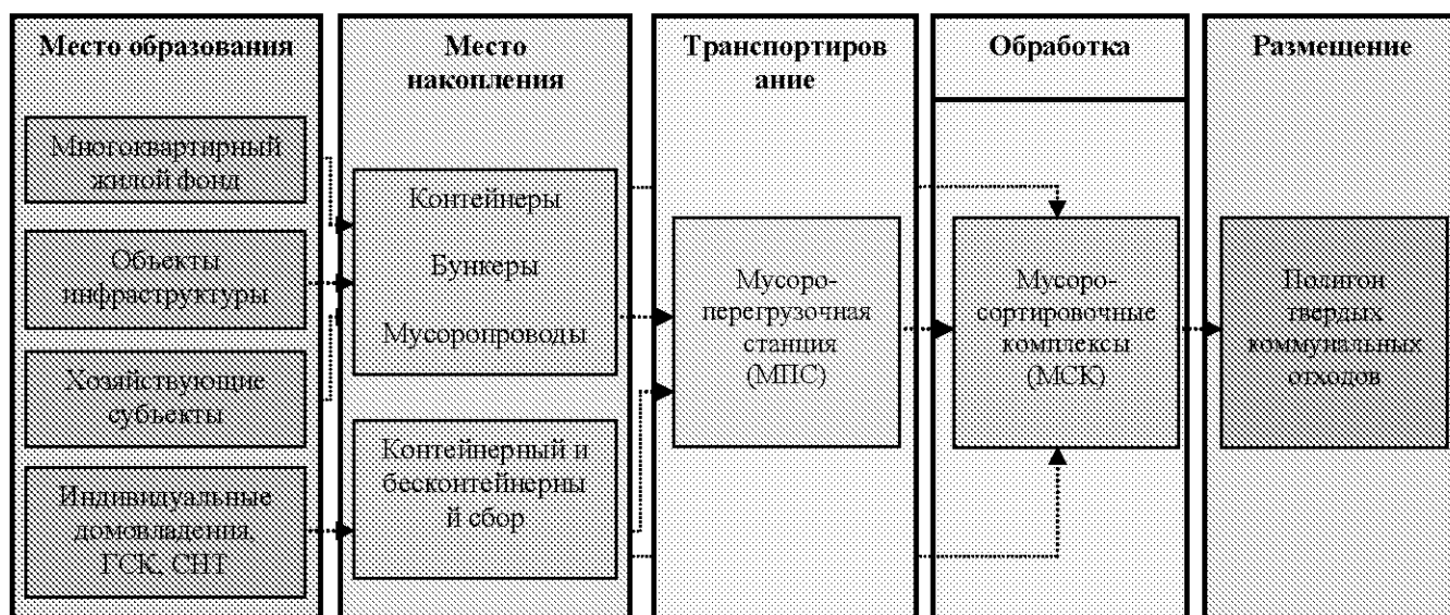
Рисунок 7.7.2 - Схема движения твердых коммунальных отходов на территории Нижегородской области
