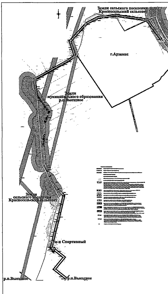
Чертеж планировки и межевания территории
