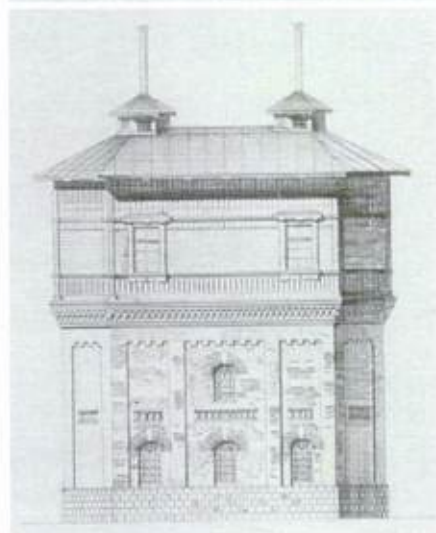
фасады водоёмного здания на 2 бака, 1902-1905 гг.
