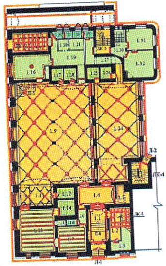
План 1 этажа
