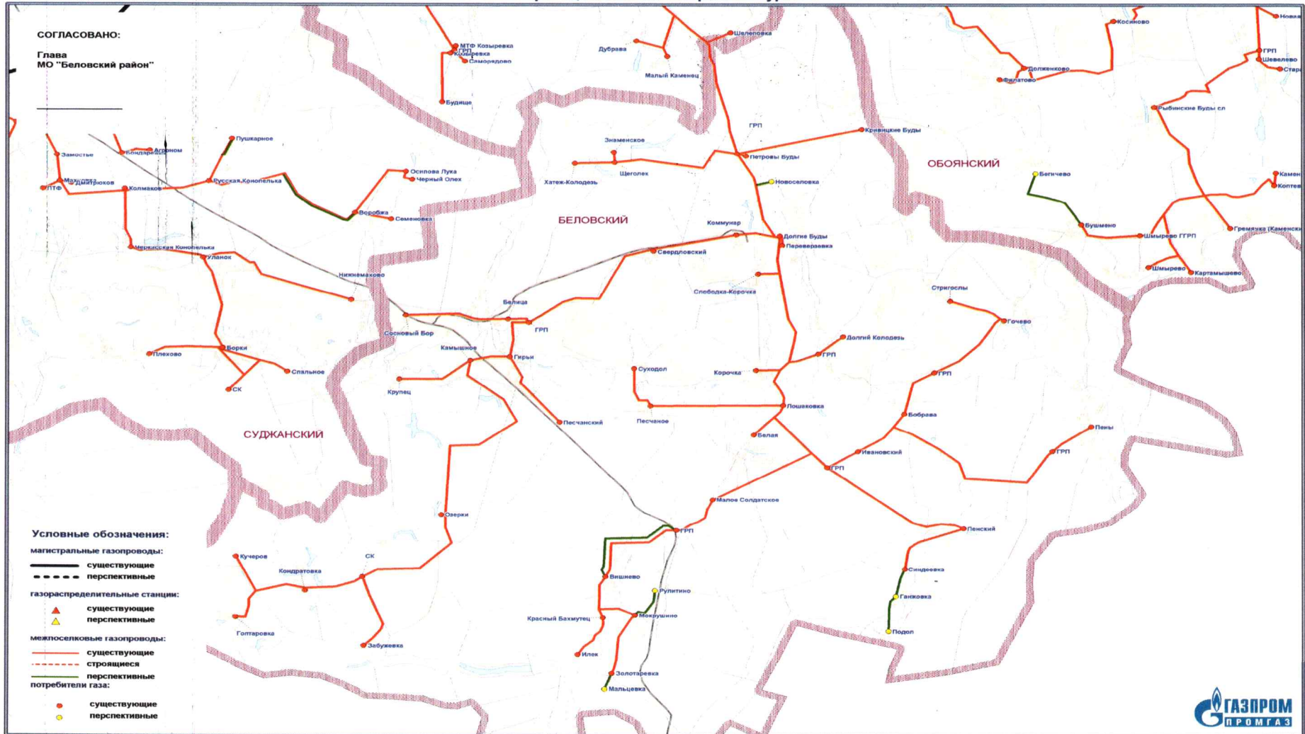
Схема газоснабжения и газификации Беловского района Курской области
