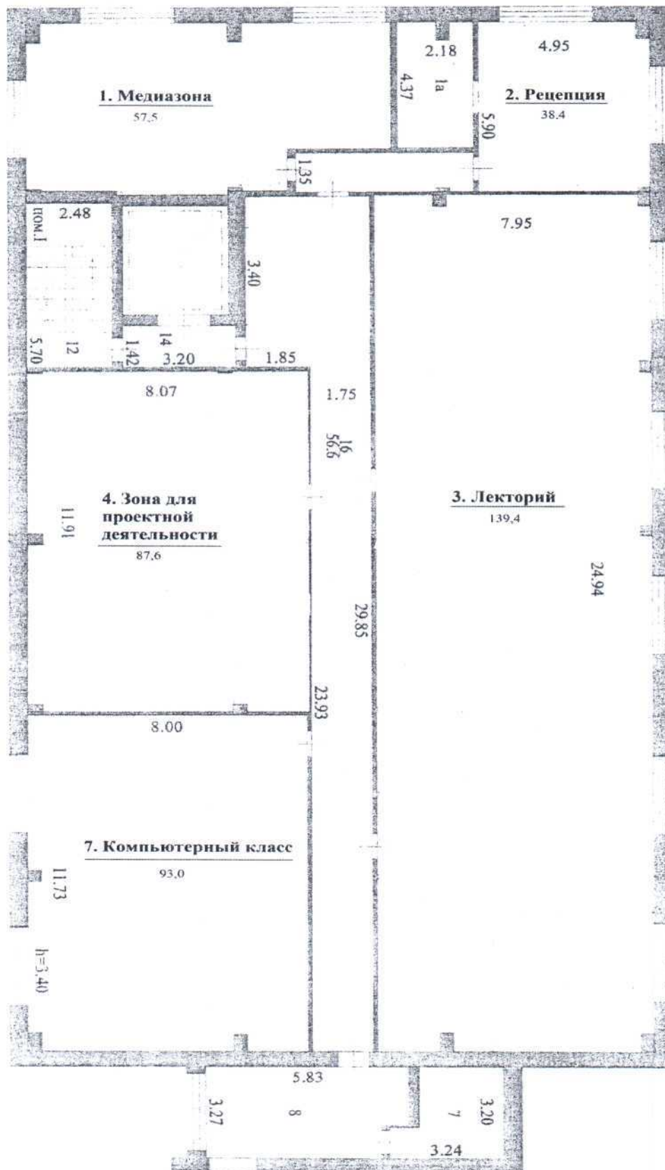
Рис.1 Зонирование. Эмпликация помещения ЦОПП (правое крыло)
