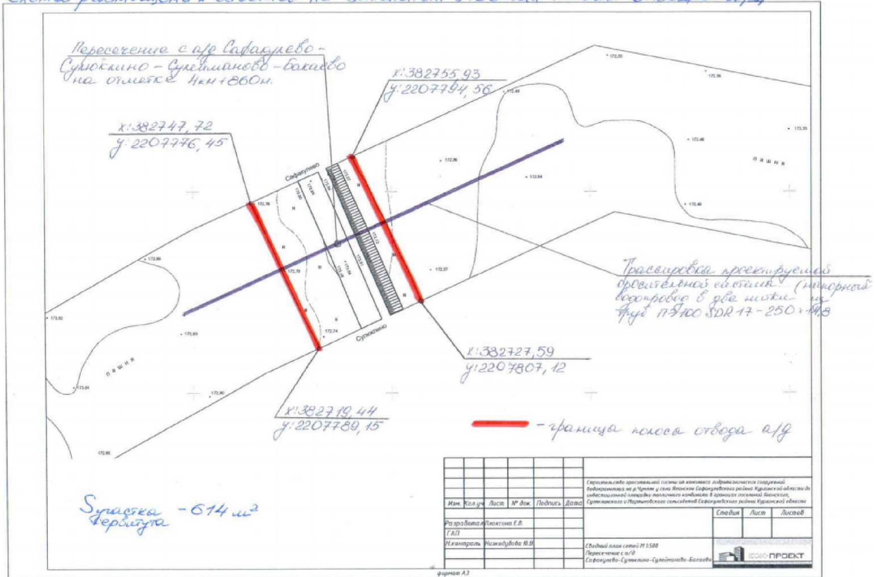
Схема размещения объекта на земельных участках полосы отвода а/д
