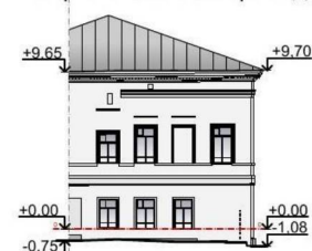
Северо-восточный фасад
