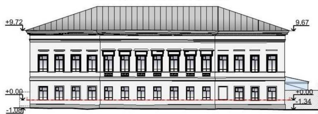
Юго-восточный фасад
