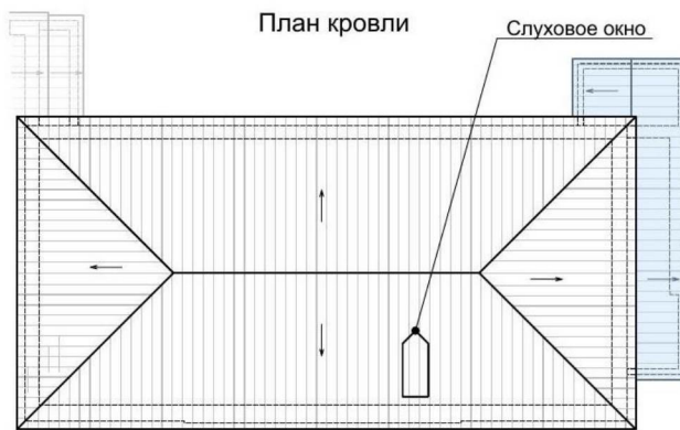
План кровли
