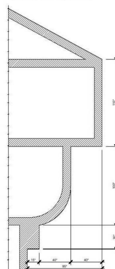
Шаблон карниза
