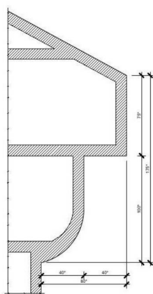
Шаблон карниза
