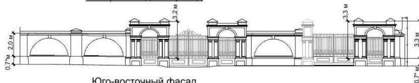
Юго-восточный фасад
