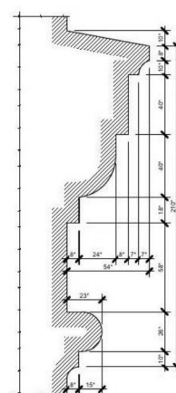
Шаблон капители
