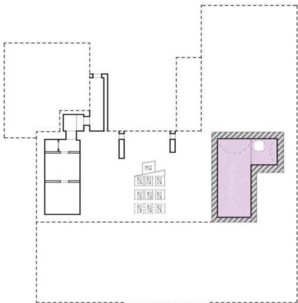
План подвала
