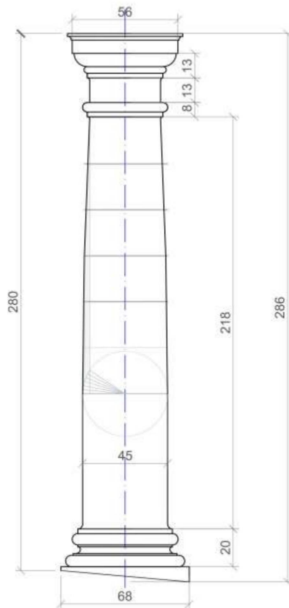
Колонна тосканского портика Рисунок 4
