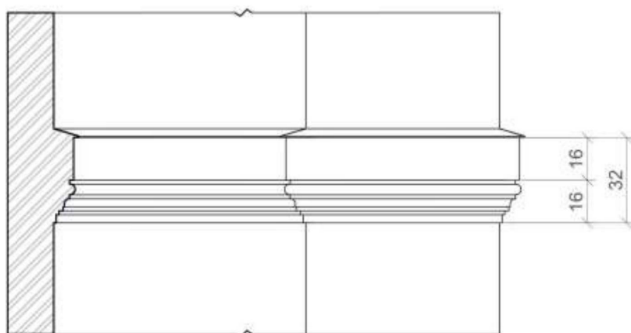
Фрагмент межэтажного пояса. Рисунок 3
