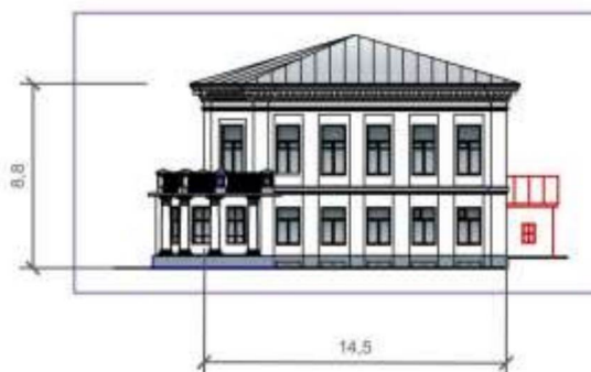
Юго-восточный фасад
