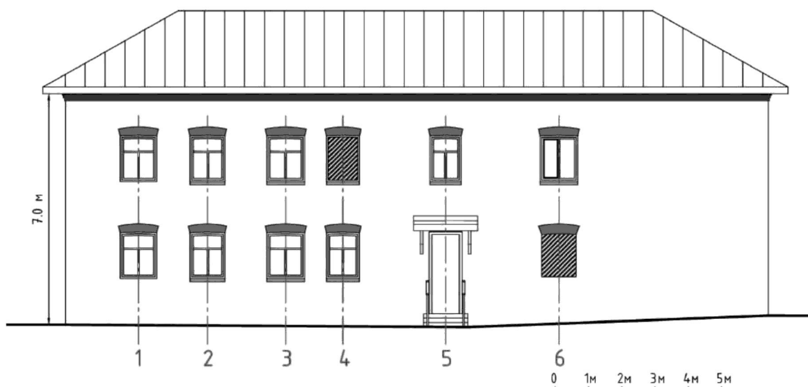
Членение фасадов. Юго-западный фасад
