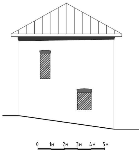
Северо-западный фасад
