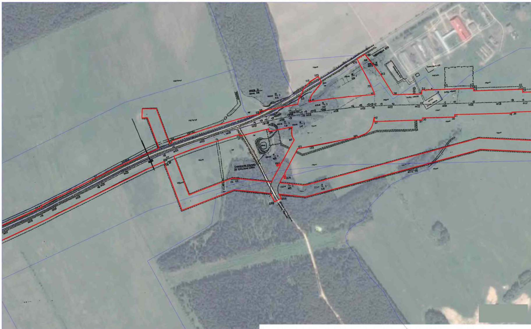
СХЕМА РАСПОЛОЖЕНИЯ ГРАНИЦ ПОСТОЯННОЙ ПОЛОСЫ ОТВОДА АВТОМОБИЛЬНОЙ ДОРОГИ (ПРЕДПОЛАГАЕМАЯ ЗОНА РЕЗЕРВИРОВАНИЯ)
