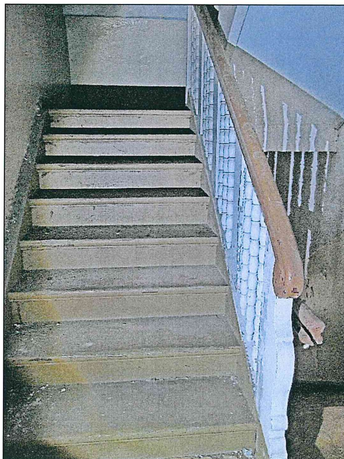
Фото 79. Третий этаж. Конструкции межэтажной лестницы.
