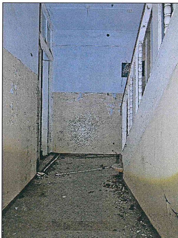
Фото 57. Первый этаж. Конструкции стен, перекрытий. Конструкции пола лестничной клетки. Дверной проем входа во внутренние помещения первого этажа.
