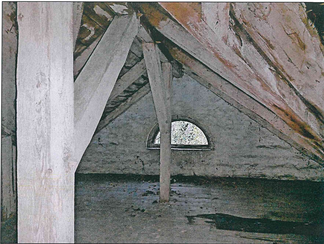
Фото 84. Чердак. Конструкции стропильной системы крыши. Конструкции оконных проемов.
