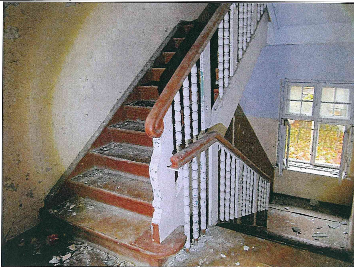
Фото 71. Второй этаж. Конструкции межэтажной лестницы.
