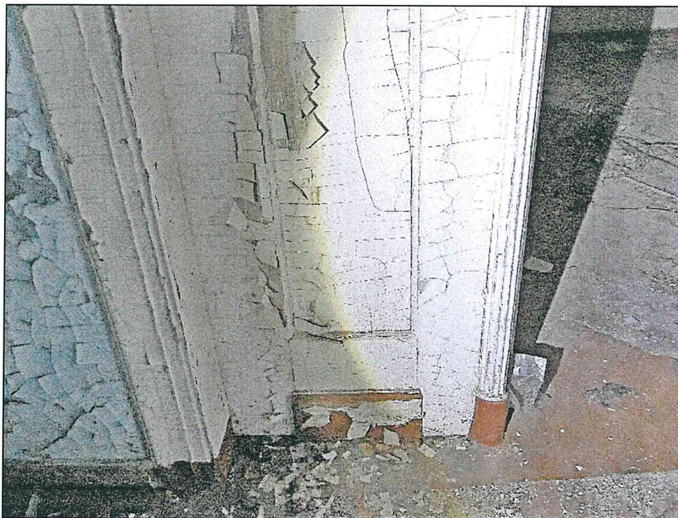
Фото 78. Третий этаж. Межкомнатный дверной проем. Конструкция дверного заполнения.
