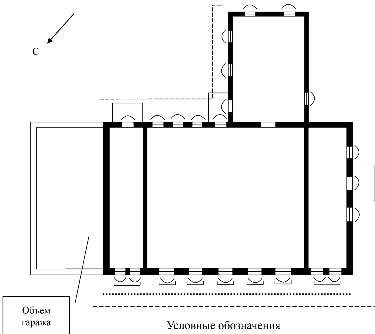
Схема обозначения предмета охраны (ценных элементов) в уровне первого этажа Доходного дома
