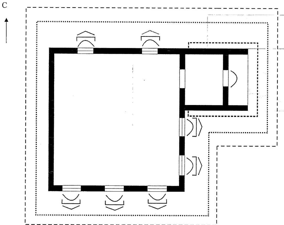
Схема обозначения предмета охраны
