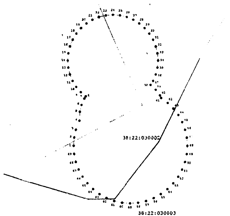
План границ объекта Второй пояс зоны санитарной охраны проектируемого водозабора на участке "Светловский 51"
