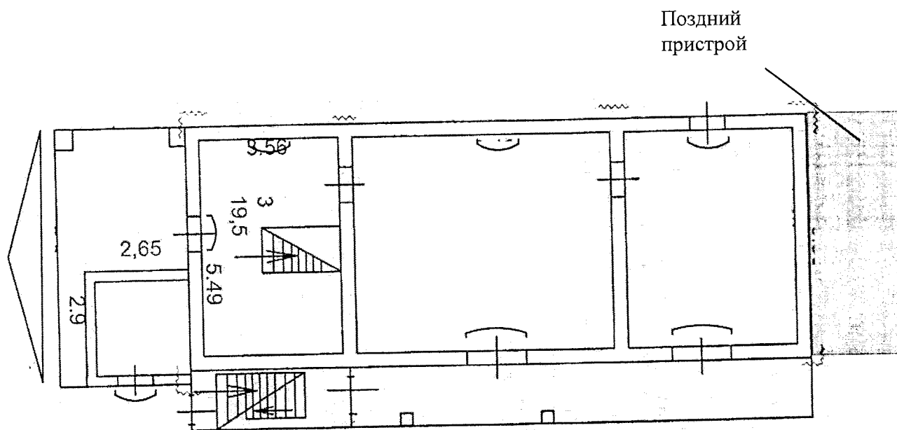
Схема расположения предмета охраны (ценных элементов) 1 этаж
