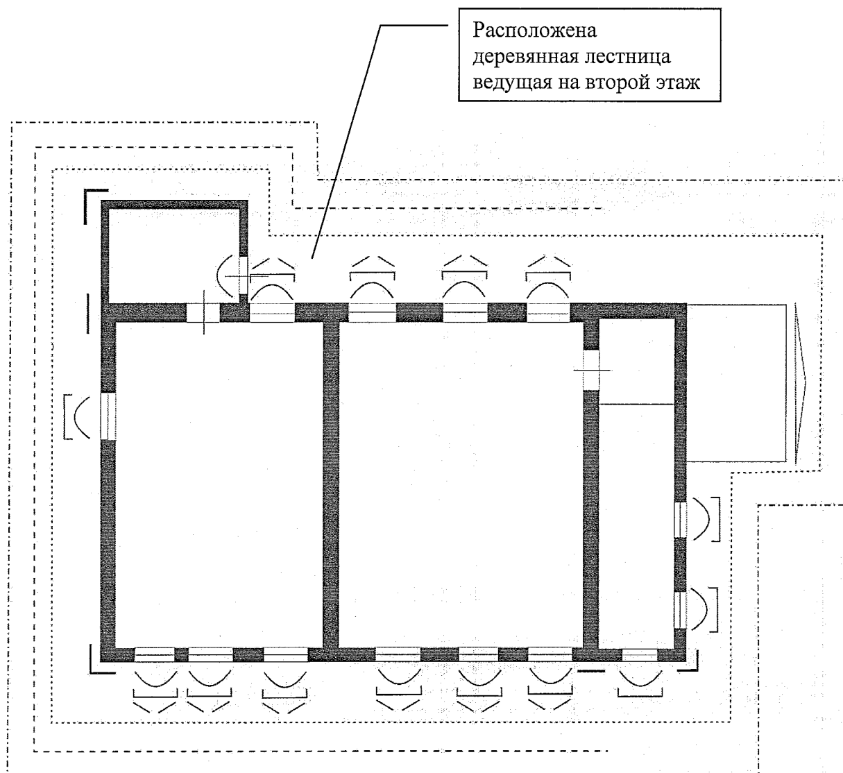
План 2 этажа
