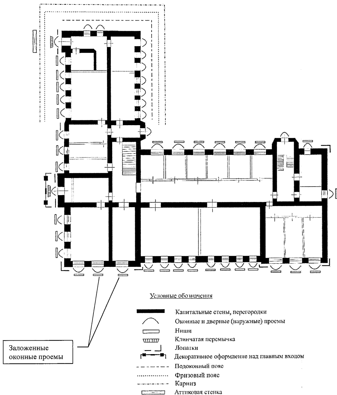
Схема 1 этажа
