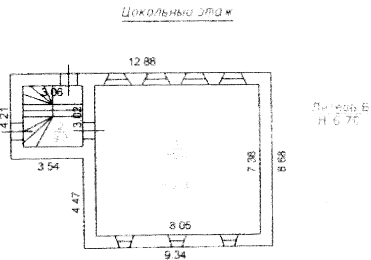
Лит. Б. Поэтажный план здания от 21.11.2011 г.
