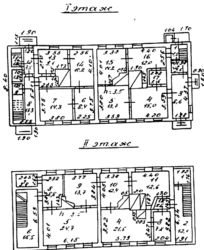
Рис.2 - поэтажный план здания лит. А 1987г.
