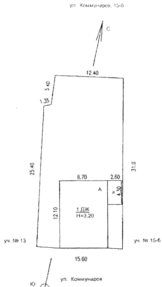
Рис. 2 - Ситуационный план, 2013 г.
