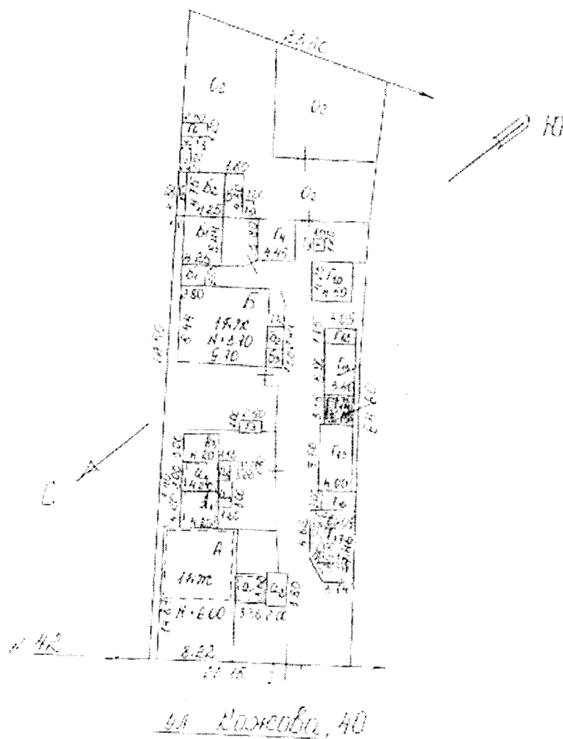
Рис. 1 – Генеральный план
