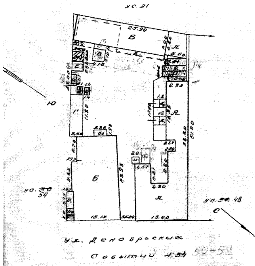
Рис.1 - Ген. план от 27.06.1961г. с корректировкой на 28.06.1983 г.
