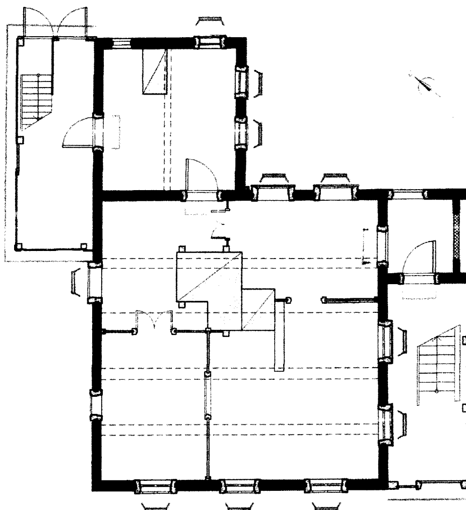
План 1-го этажа. М 1:50
