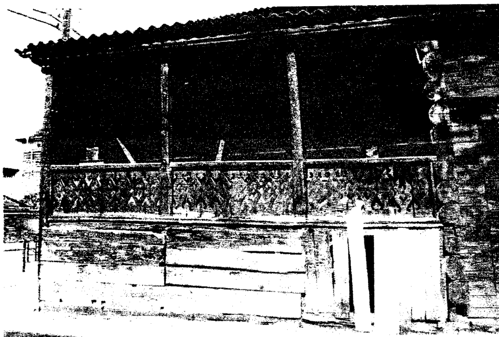
Фото 14. Галерея.
