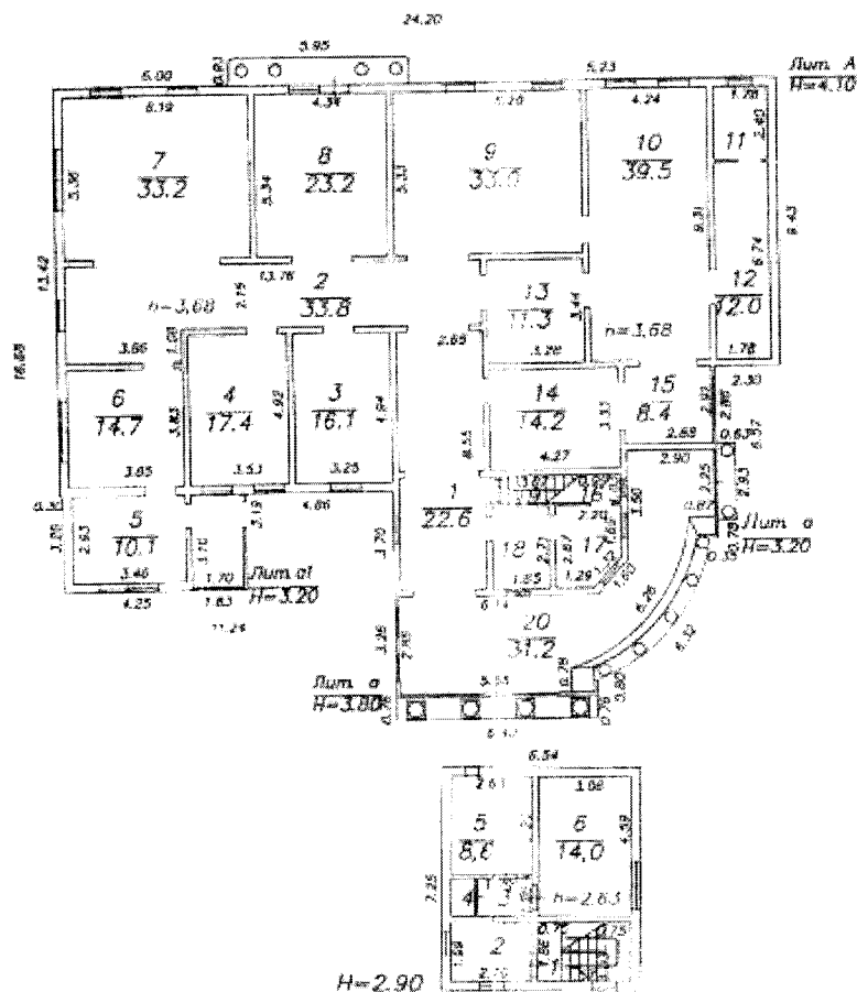
Рис. 2 - Планы 1-го 2-го этажей дома по ул. Мира, 20. (инвентаризация БТИ 2009 г.)
