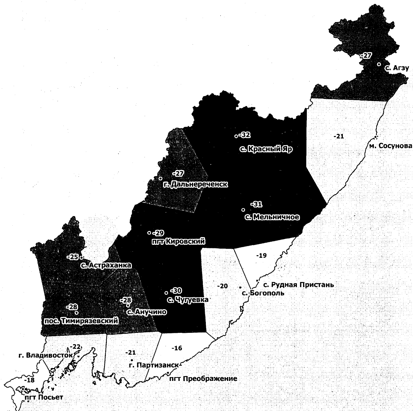
Рисунок 1 – Распределение температуры наружного воздуха наиболее холодной пятидневки на территории Приморского края по данным метеорологическим станциям, °С
