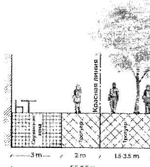
Пешеходный модуль тип 2
