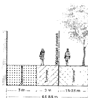
Остановка ОТ с полосой озеленения
